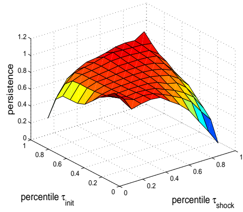
(d) Bandwidth=.4
